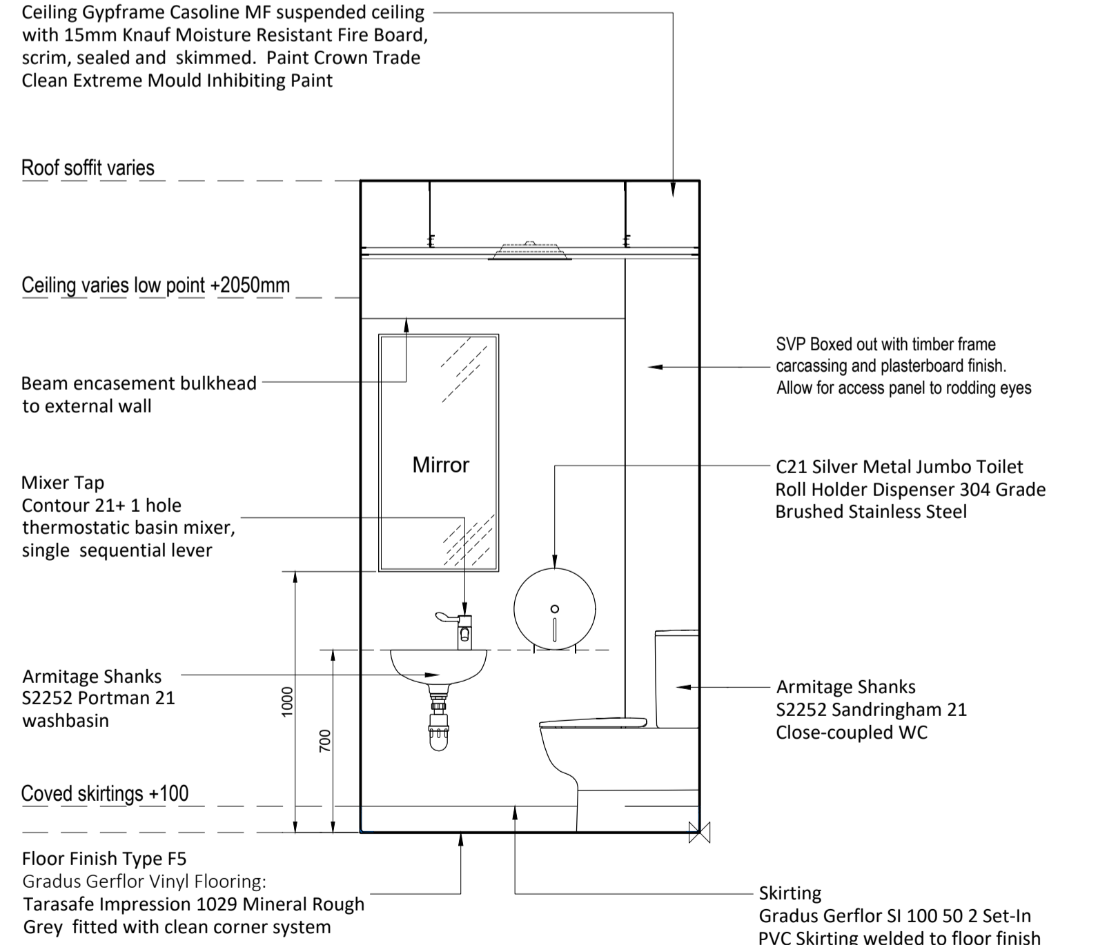
ELEVATION D2
