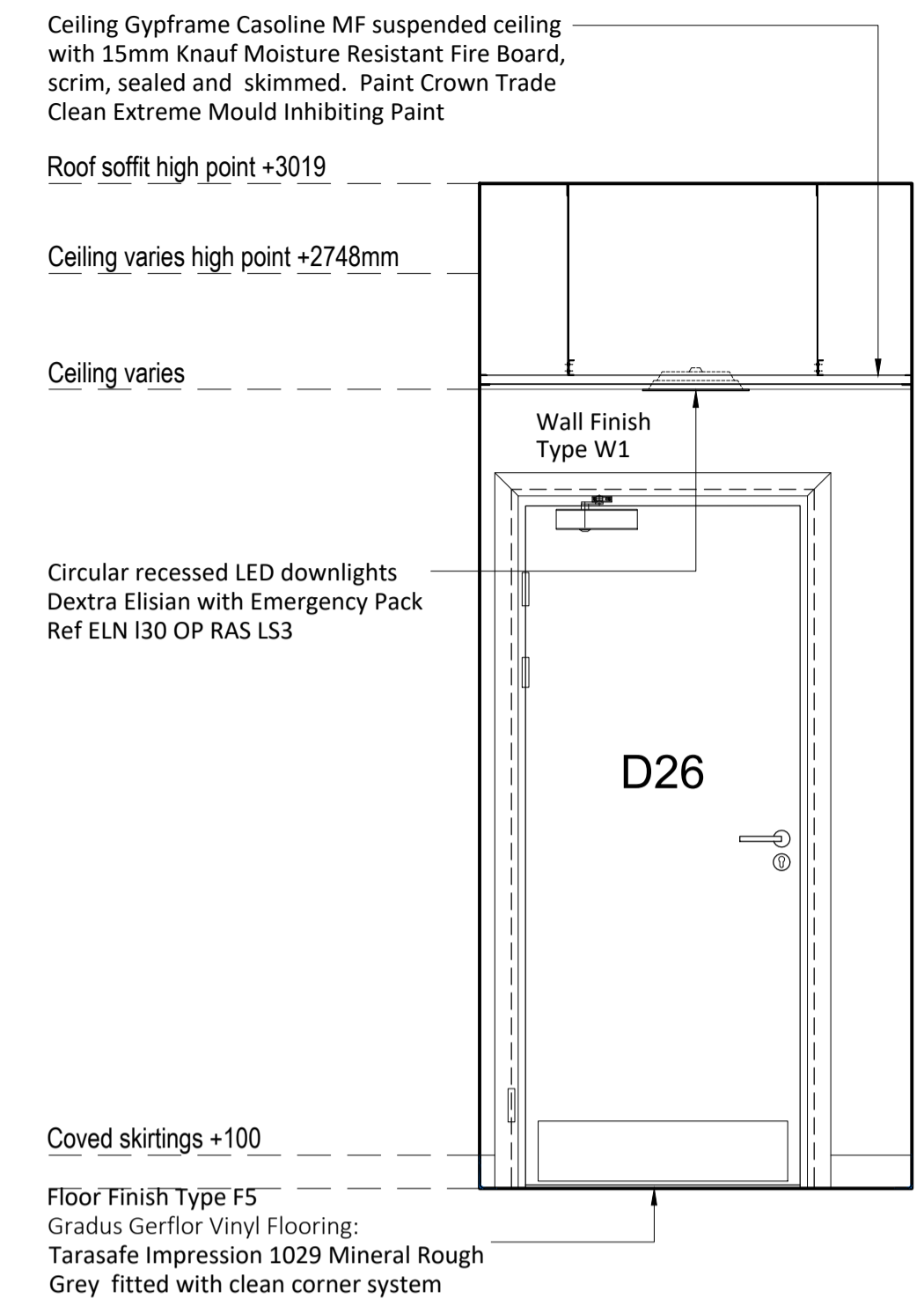
ELEVATION B
