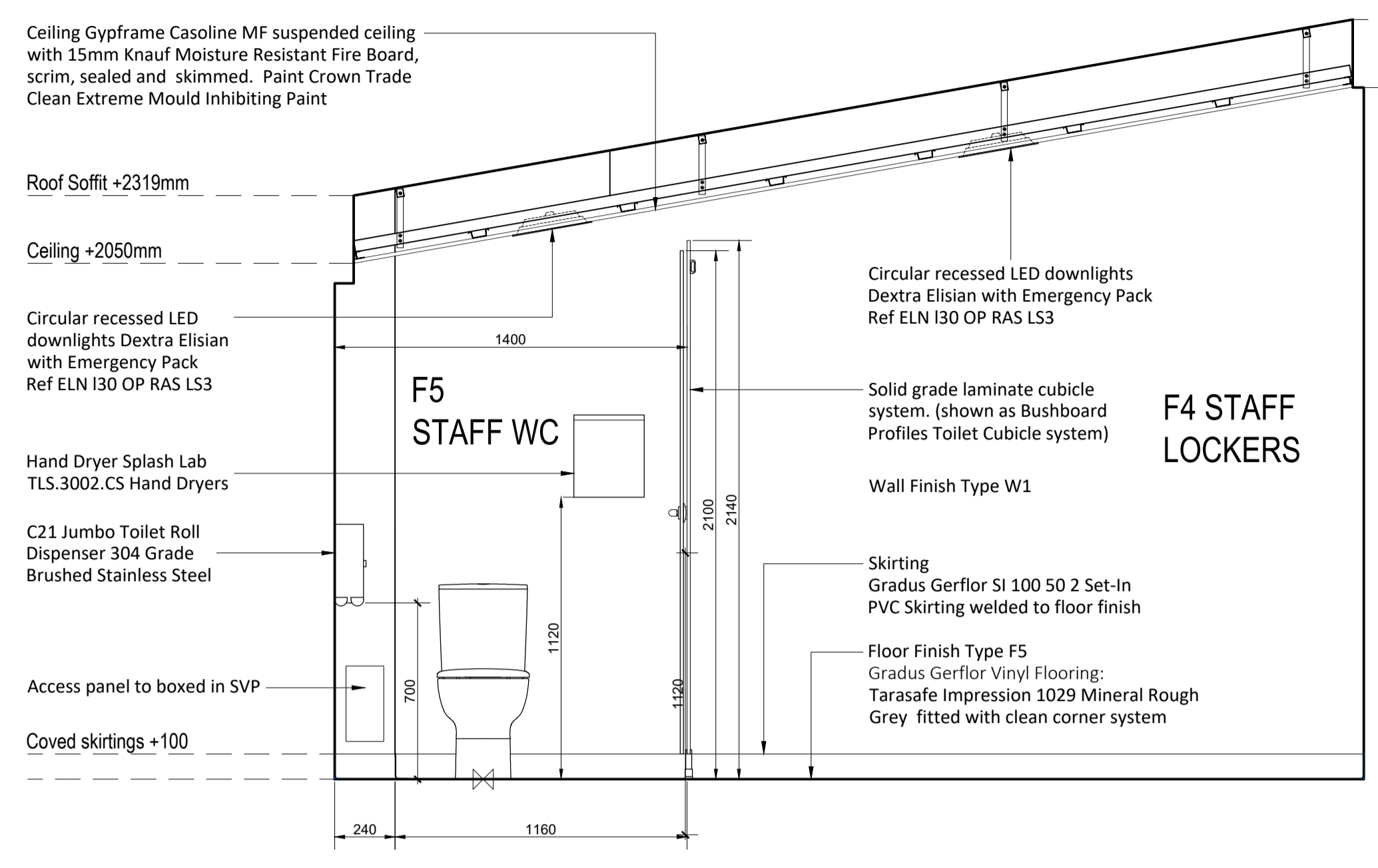
ELEVATION A
