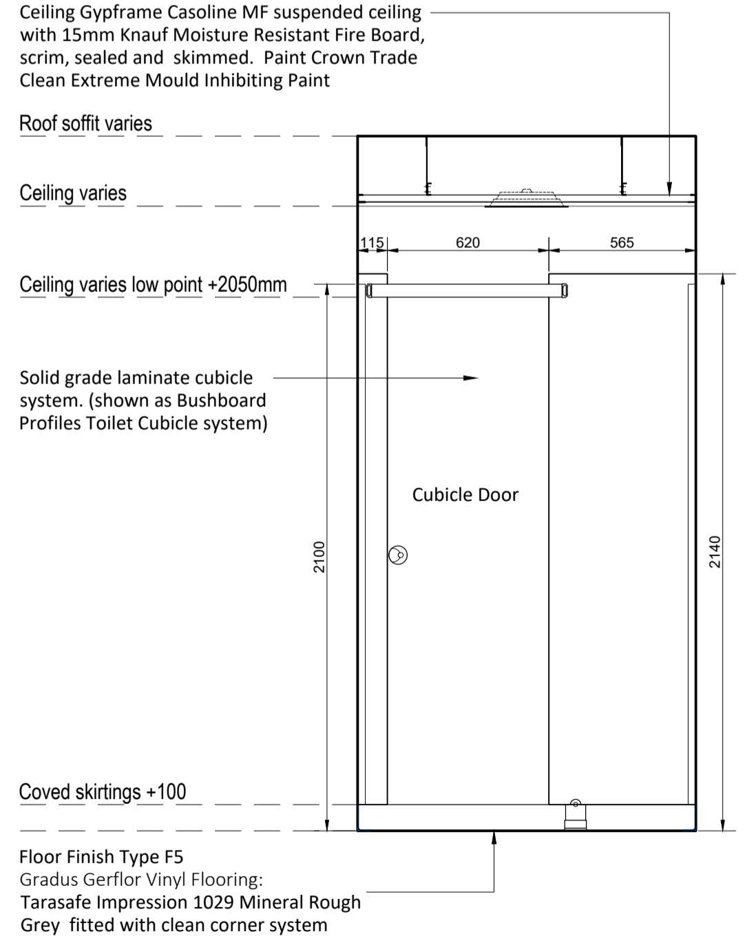
ELEVATION D1
